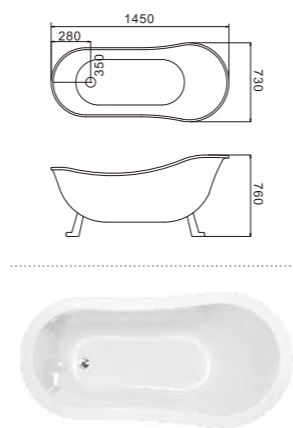
C-3253 Size:730x1450x760/mm
